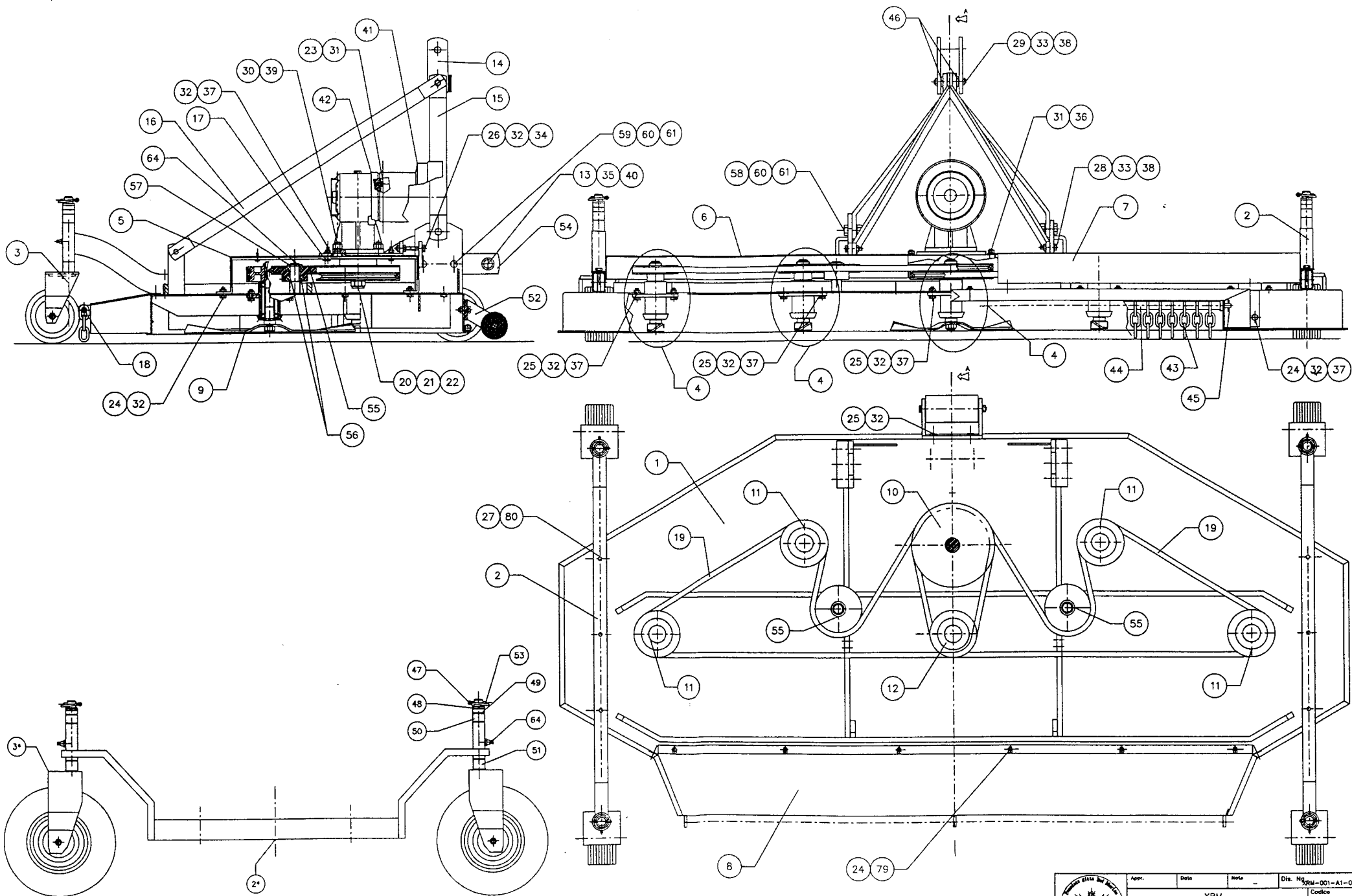
PORTARUOTE E GRUPPO RUOTE PER VERSIONE CON RUOTE PNEUMATICHE
